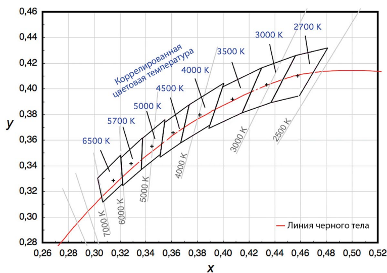
Рис. 2. Графическое представление цветных показателей твердых источников света на диаграмме x, y CIE 1931
